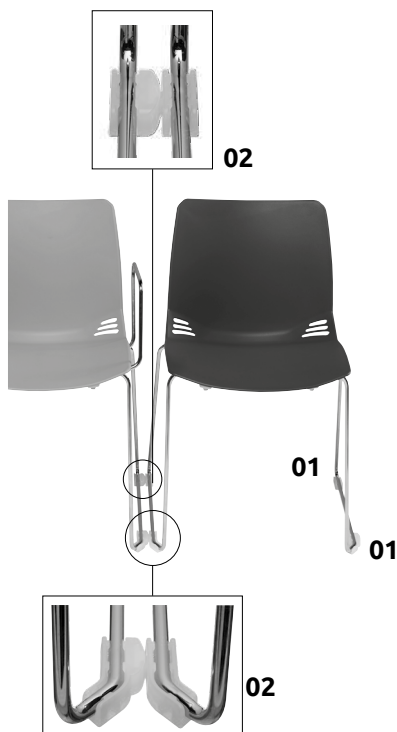
Versione sedie senza tavoletta Version for chairs without tablet (02+01)
